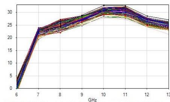
КПД по добавленной мощности (PAE P1dB), %
