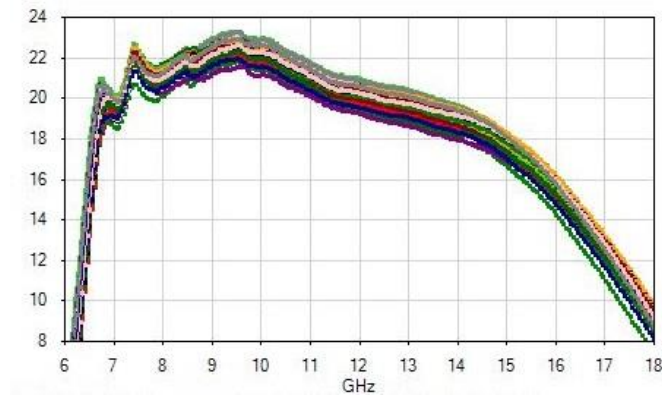
Возвратные потери по выходу (S22), дБ
