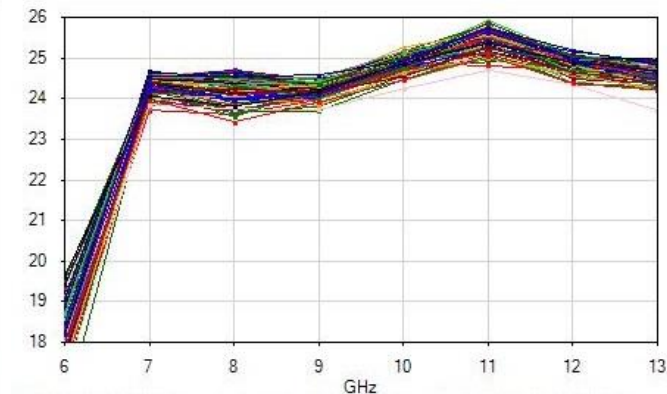
Выходная мощность (P1dB), дБм
