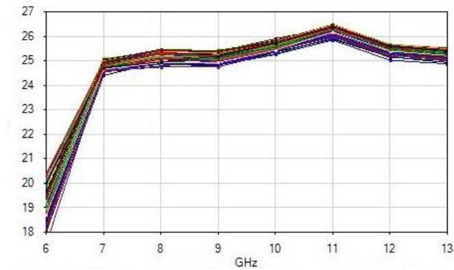
Выходная мощность (P3dB), дБм
